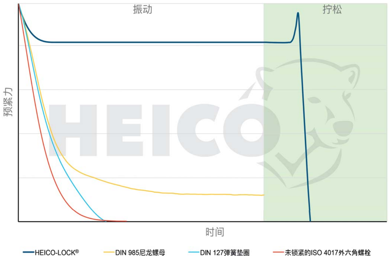
图：根据DIN 65151/DIN 25201-4标准进行的振动测试，演示预紧力丢失过程
